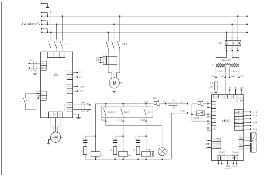
Bild 2.6 Elektro-Schaltplan DV75-90
