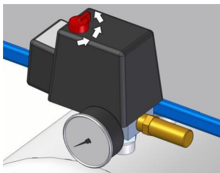
Рис. 35: Выключение компрессора
