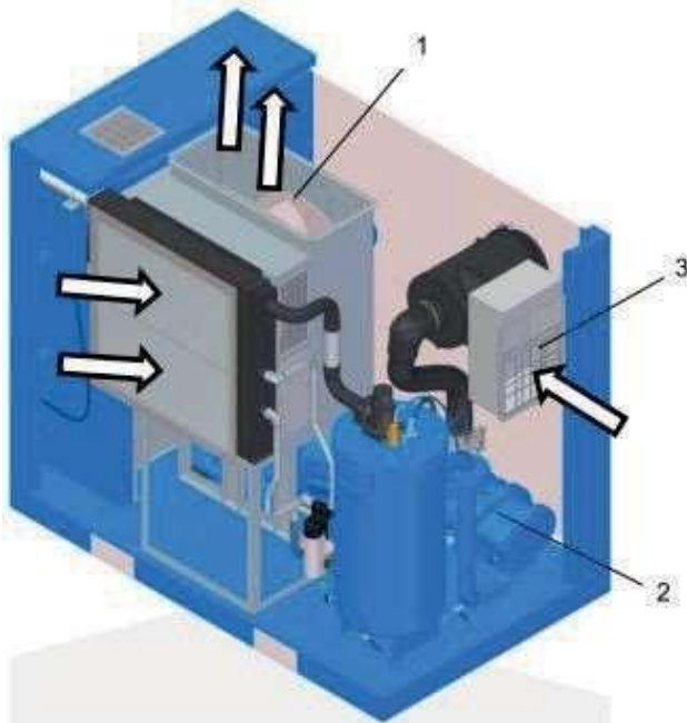
Рис. 15: Вентилятор охлаждения и воздушный фильтр
