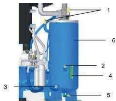
Рис. 8: Маслобак-сепаратор компрессорного масла с предохранительным клапаном
