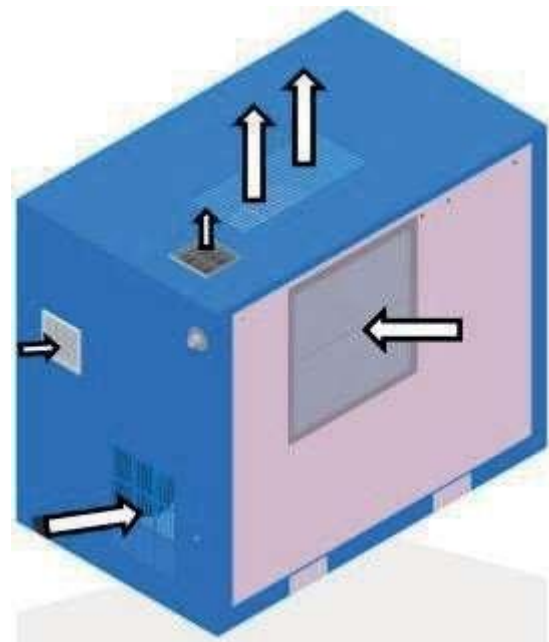
Рис. 27: Обзорная схема движения воздуха
