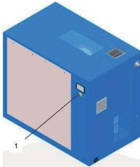
Рис. 18: Кнопка аварийного выключения (поз. 1) на винтовом компрессоре GEAR XP 75 – 90 / VARIABLE XP 75 – 90
