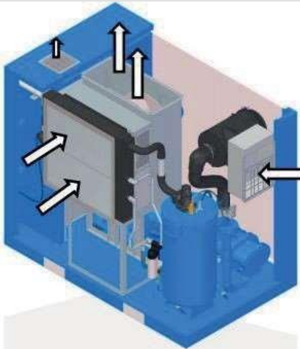
Рис. 26: Винтовой компрессор GEAR XP 45 – 90, VARIABLE XP 45 – 90
