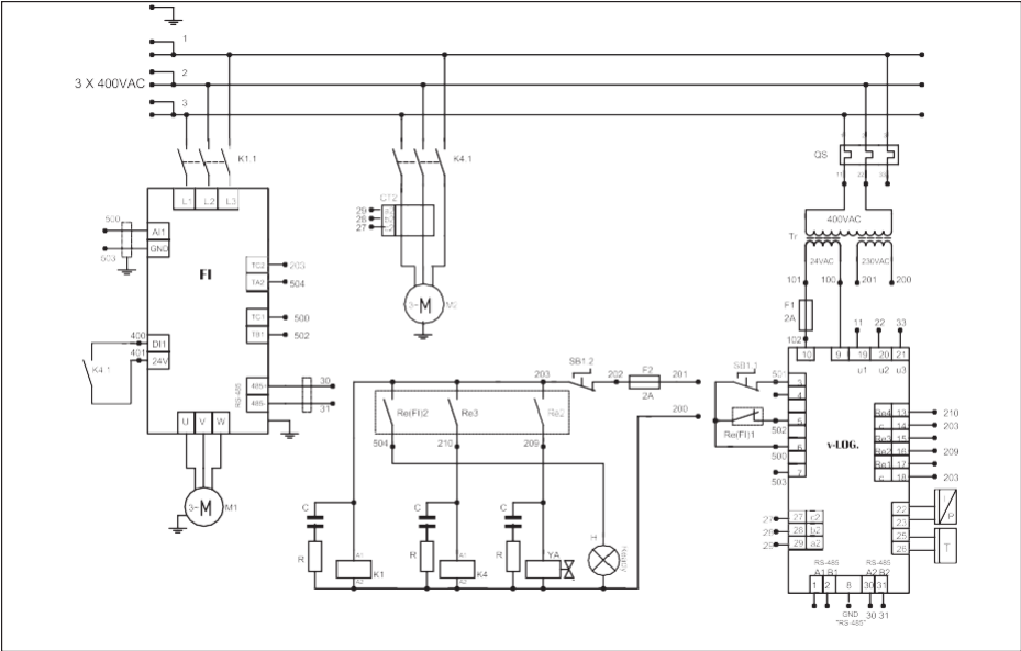
Bild 2.6 Elektro-Schaltplan DV75-90
