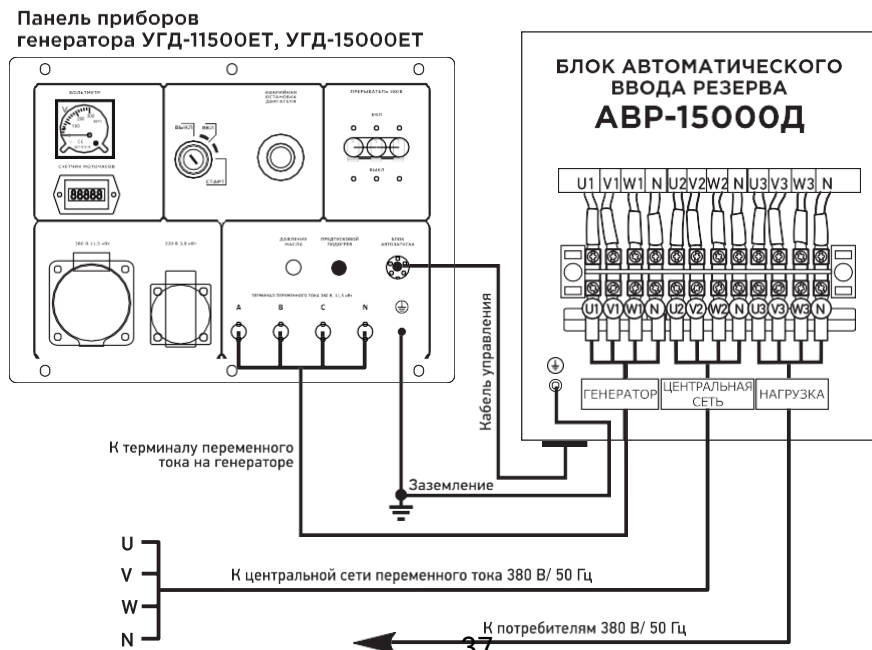
Рис. 23. Схема подключения блока АВР-15000Д к трехфазному генератору 380В
