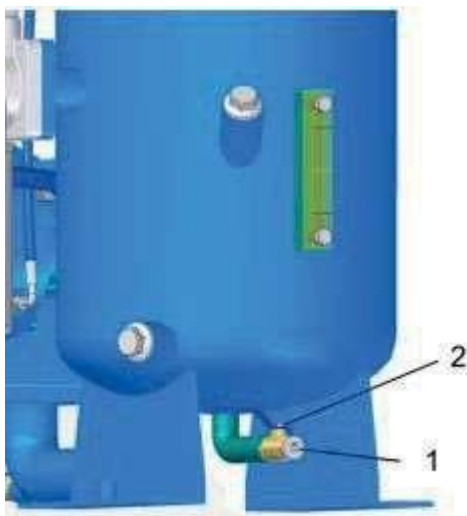
Рис. 35: Отверстие для слива масла
