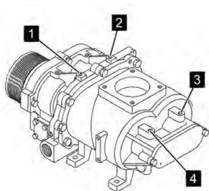
Рис. 55: Точки смазки для типа 15 – 30
